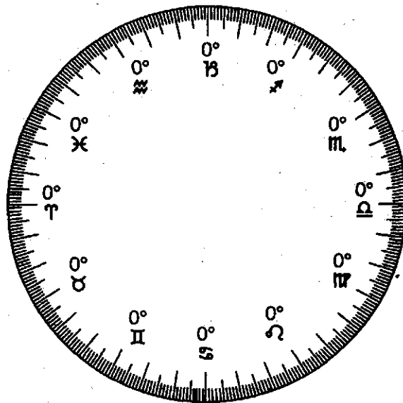
Рис. 1.3 Зодиакальный круг
